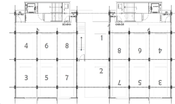
PLANTA TIPO. NIVEL DE ACCESO
